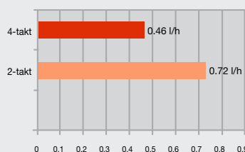
Brandstofverbruik (liter/uur)
